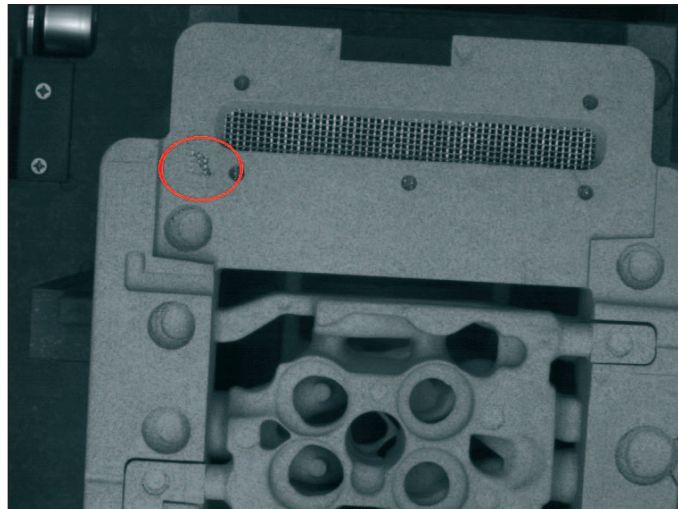
Abb. 2: Bei der Oberflächenprüfung stellt das Bildverarbeitungssystem einen Fehler fest: Die Netzeinlage zum Schutz der Kernvertiefung ragt aus der Kernoberfläche heraus.
