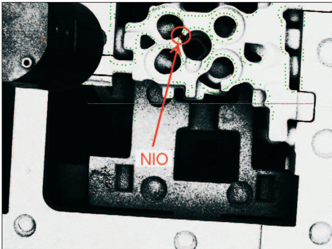
Abb. 1: Prüfung auf Formausbrüche an einem Kernpaket für einen Mercedes-Benz-5-Zylinder-Motor. Durch das Vergleichsbild erkennt die Software verschiedene Geometriefehler (rot gekennzeichnet).
